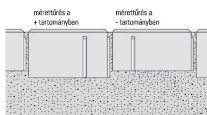
22. ábra: A térkövek helyzete tömörítés után (a méretbeli különbségek az ágyzatban egyenlítődnek ki)
