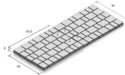
26. ábra: Viato Mistro – rakásminta gépi rakáshoz (vegyes méretek, futósoros)
