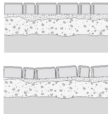
14. ábra: Helytelen rakásmód: a térkő és a távtartók összeérnek
